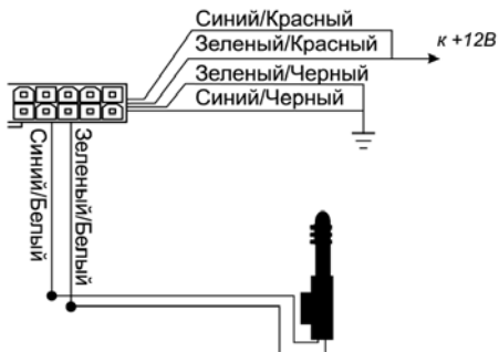
Схема 6. Установка дополнительных электродвигателей
